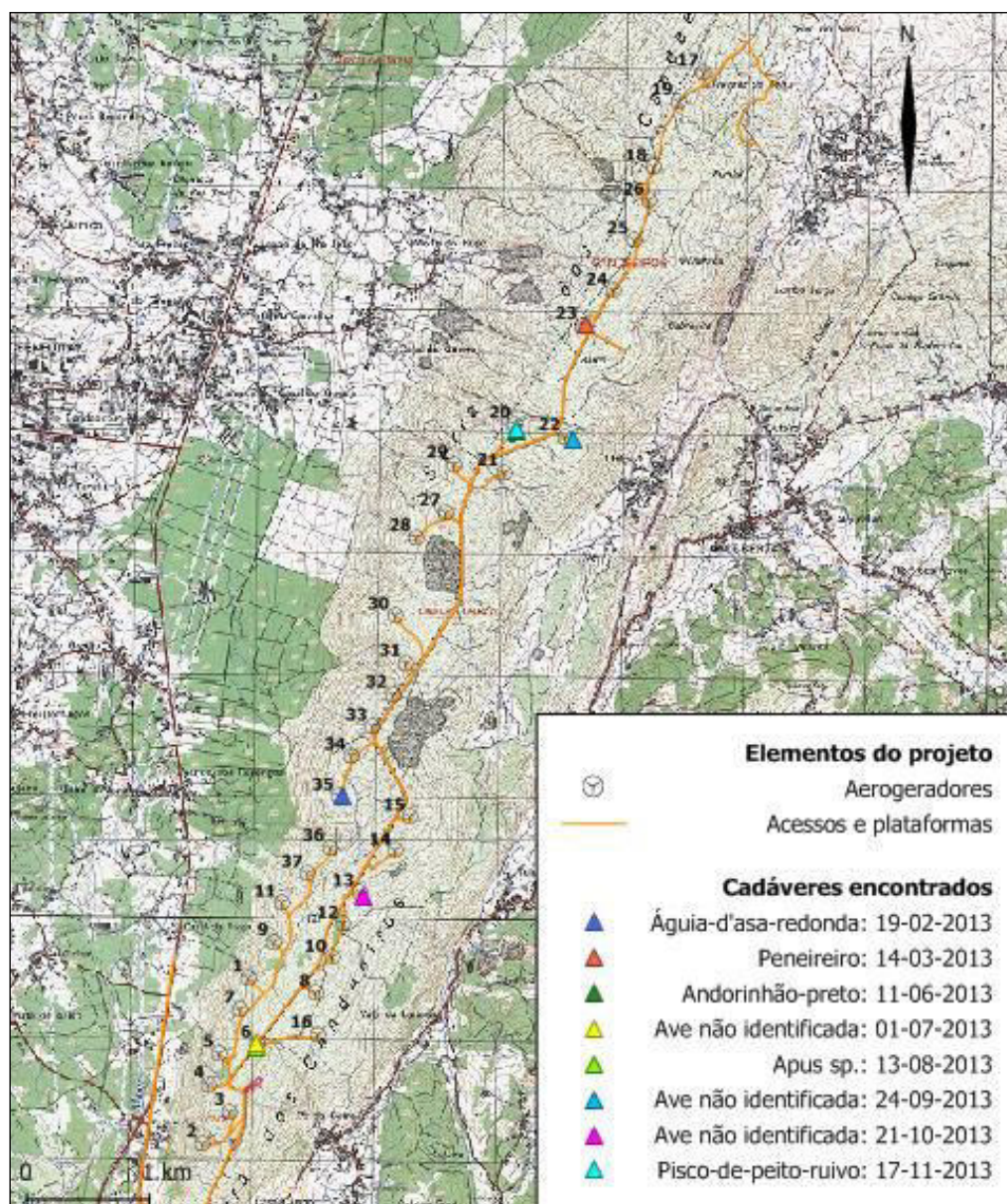
Figura 7 – Localização dos indícios de mortalidade encontrados durante as prospeções de cadáveres efetuadas em redor dos aerogeradores do Parque Eólico da Serra de Candeeiros em 2013.
